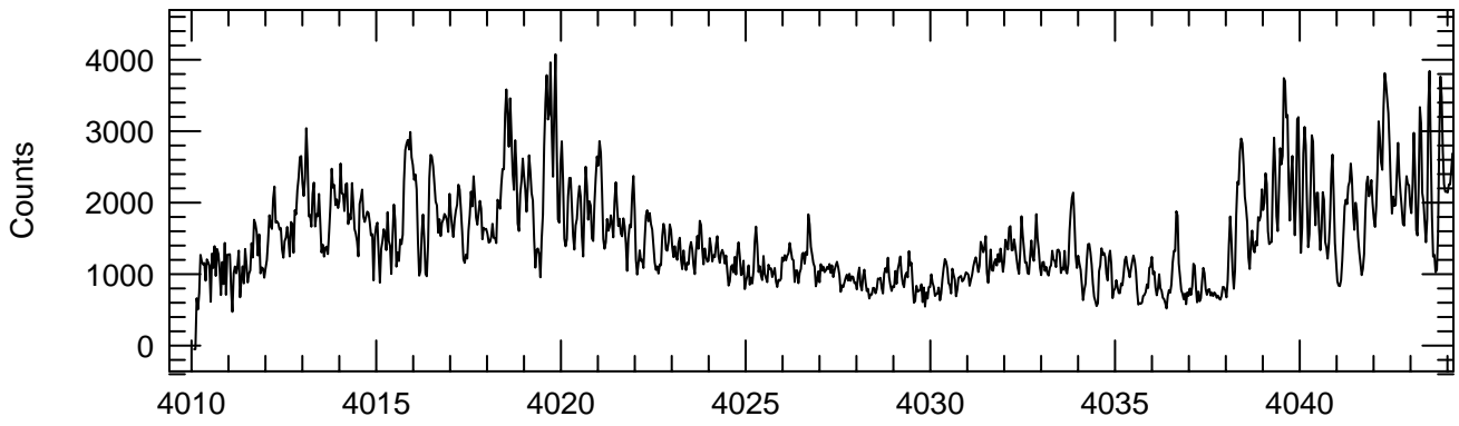
122P/de Vico -- RV23257 (optocenter)
